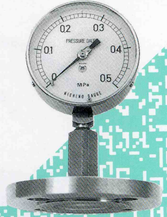
フランジ式 FW
