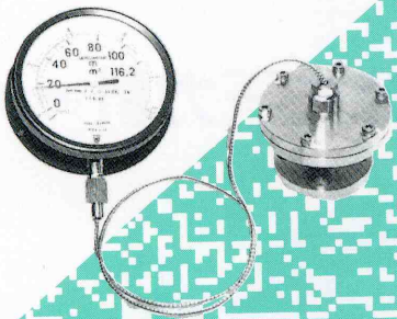
隔測式タンク用 D-130 (液面計)
